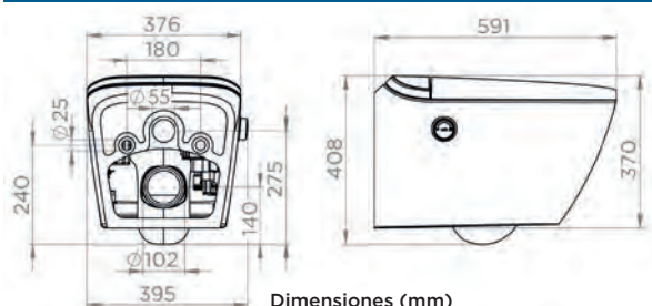
Dimensiones (mm)
