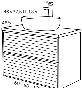
Mueble 12010 Lavabo sobreencimera LINE + Tapa TEXTURA 21680 (A) (A) Encimera con agujeros para lavabo y grifo
