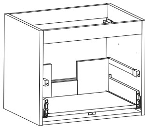
Modelo 12012 un Frente con un Cajón inferior
