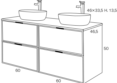
Mueble 16010 x 2 ud Lavabo sobreencimera LINE x 2 und + Tapa PL 21683 (A) (A) Encimera con agujeros para lavabo y grifo
