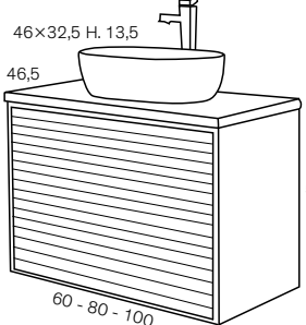
Mueble 12012 Lavabo sobreencimera LINE + Tapa TEXTURA 21680 (A) (A) Encimera con agujeros para lavabo y grifo
