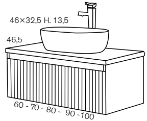
Mueble 81011 Lavabo sobreencimera LINE + Tapa PL 21680 (A) (A) Encimera con agujeros para lavabo y grifo
